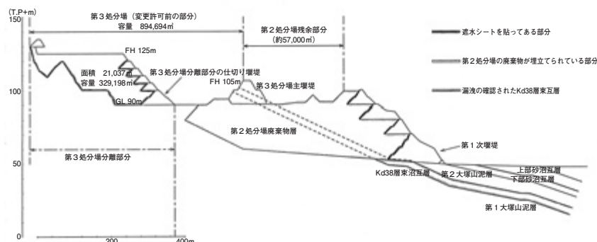
第2処分場・第3処分場断面図（イメージ図）
